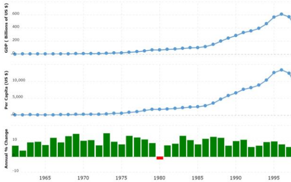
Fig. 3. GDP
